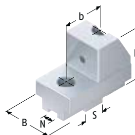
TRQK ...-2
