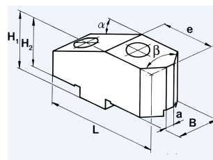
5 Gewichtserleichterung schräg und Ansrägung 60° oder 120°
