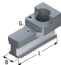
PT-FR / PT-S ...-2 - 4
