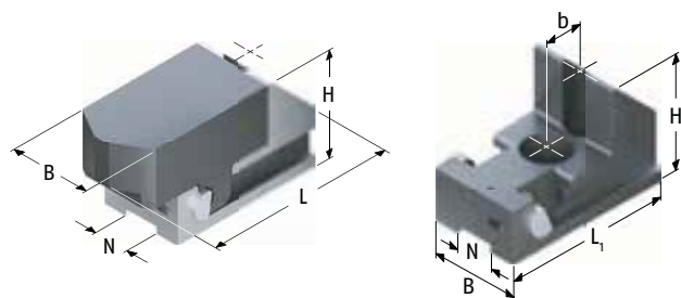
Schnellwechselbacke, komplett Quick Change Jaw, complete
