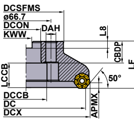
Рис.3 ø160
