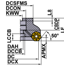
Рис.1 ø63 ø80
