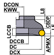
Рис.2 ø125
