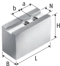
Weiche Aufsatzbacken SWB-AL Aluminium Soft Top Jaws SWB-AL Aluminium
