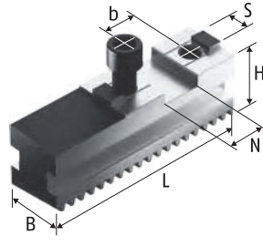
Grundbacken GBK Base Jaws GBK
