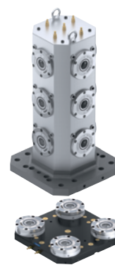
Комбинация с монтажными стойками
