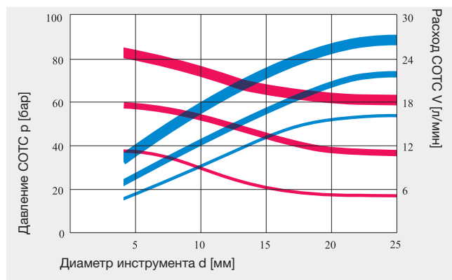
Рис. 3 : Необходимые давление и расход СОТС для обработки GG25 сверлами Ratio с прямыми канавками типа RT 150 GG.
