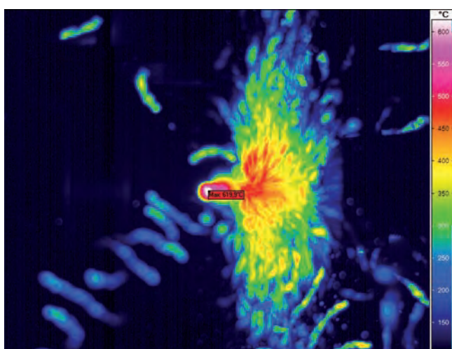
Традиционная без СОТС \vartheta_{\max}: 619^\circ\text{C}
