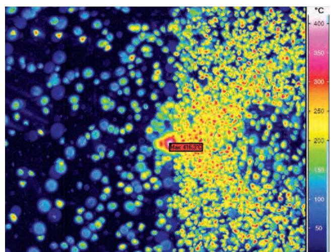
С наложением колебаний без СОТС \vartheta_{\max}: 416^\circ\text{C}
