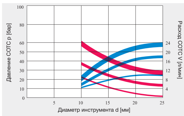
Рис. 2 : Необходимые давление и расход СОТС для сверл Ratio тип RT 80 с центральным каналом СОТС
