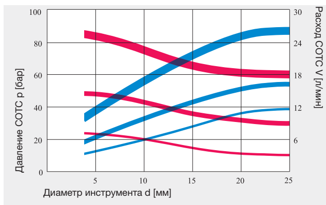
Рис. 4: Необходимые давление и расход СОТС для обработки AlSi7 сверлами Ratio с прямыми канавками, тип RT 150 GG.
